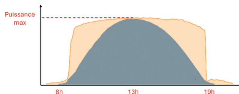
Comparatif de production entre un tracker solaire (en orange) et une installation fixe équivalente orientée sud (en bleu)
