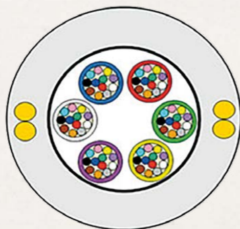
Exemple d'un câble de 72 fibres optiques
